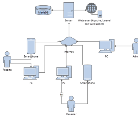
Gambar 1. Desain Arsitektural Website Kuisin
