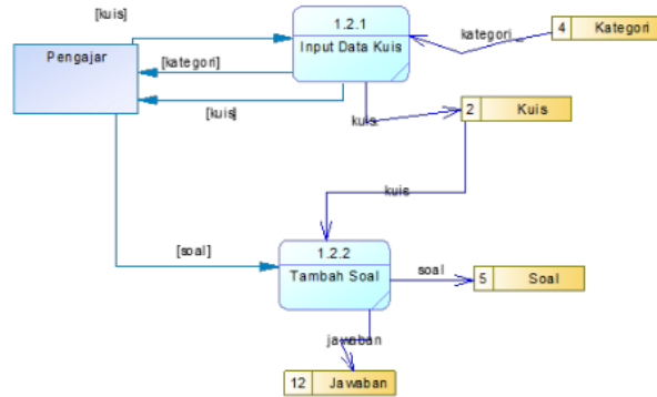
Gambar 4. DFD Level 2 Proses Pembuatan Kuis
